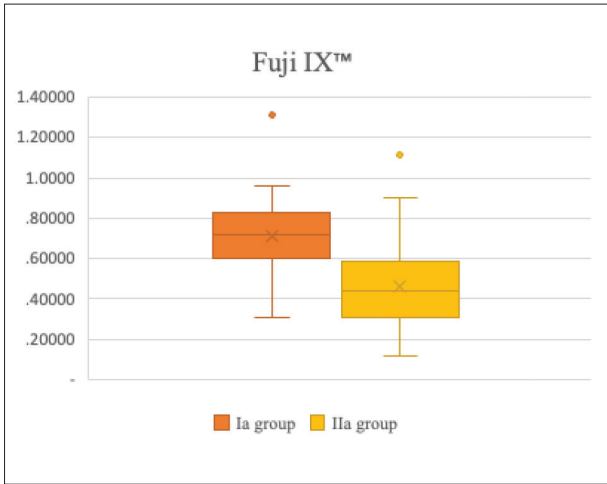
Figure 4. Crack size distribution of untreated and finished Fuji IX™ samples, expressed in µm Slika 4. Raspodela veličina pukotina na neobrađenim i obrađenim uzorcima Fuji IX™, koje su izražene u µm
